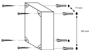
Inštalácia na stenu
