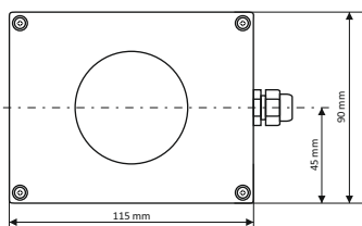
Inštalácia na stenu
